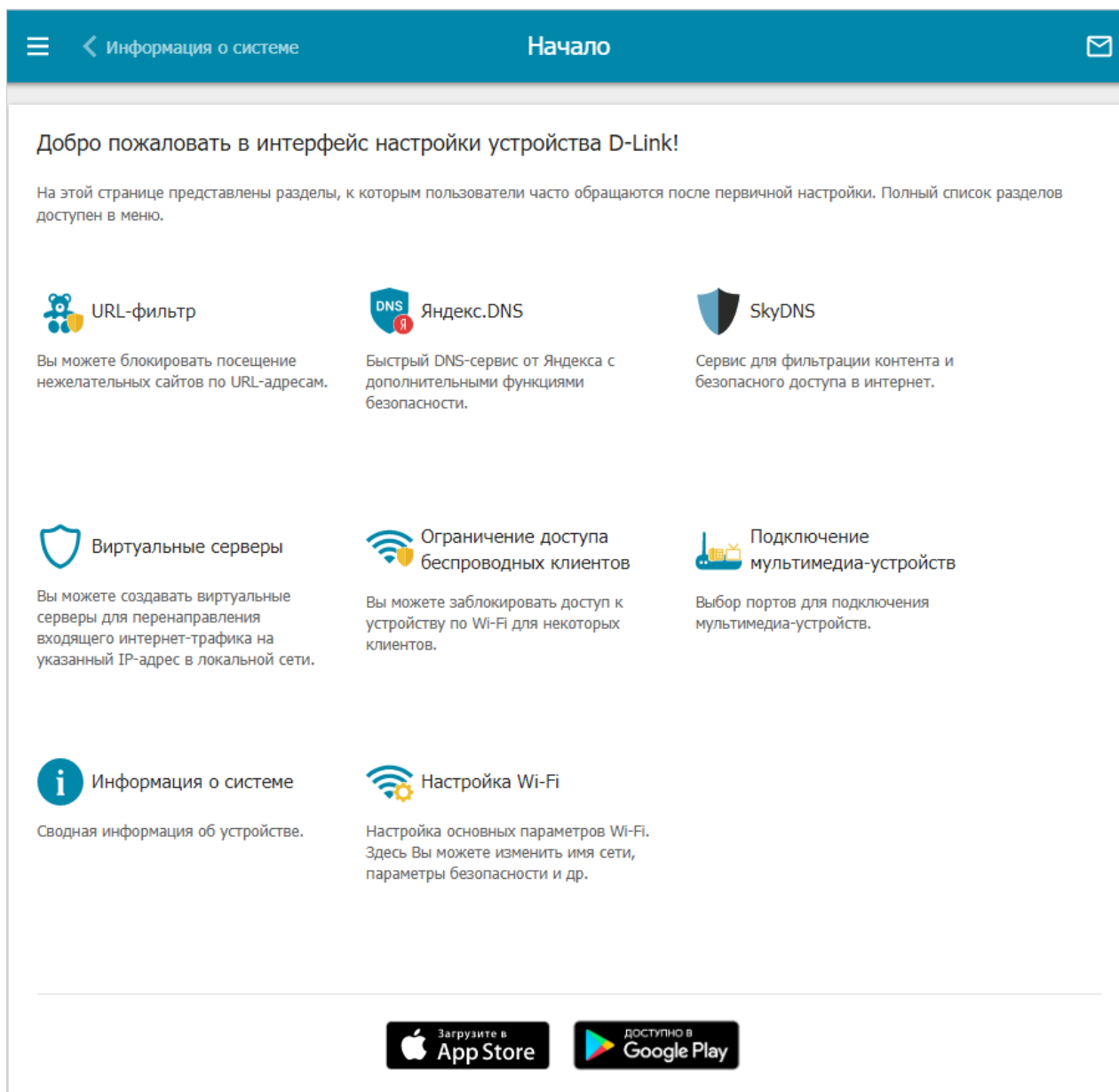
Рисунок 26. Страница Начало .
