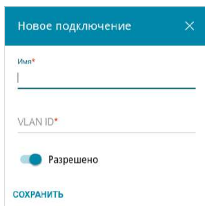
Рисунок 54. Добавление подключения.
