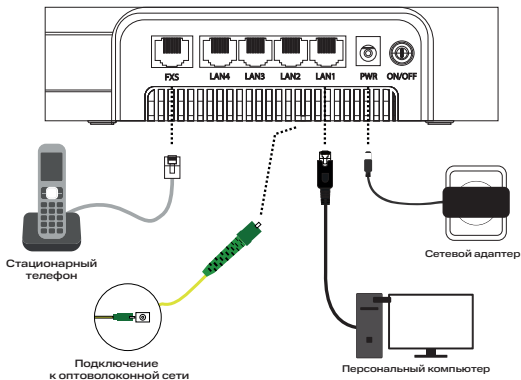
Рис. 6: Порты для подключения
